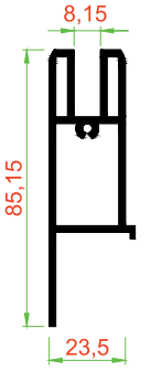
TGT-107 AÇILIR CAM BAZA (TEK CAM) 0.886 KG/M
